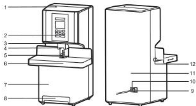
1.铝管(入料口) 2.液晶显示屏 3.防护罩 4.导电橡胶垫 5.钻刀 6.工作台面 7.前壳 8.纸筒盒 9.电源线 10.电源开关 11.后壳 12.台面固定旋钮
